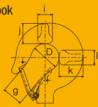
Bottom Hook
